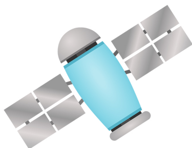
Sonda kosmiczna
