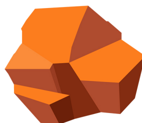
Meteoryt
