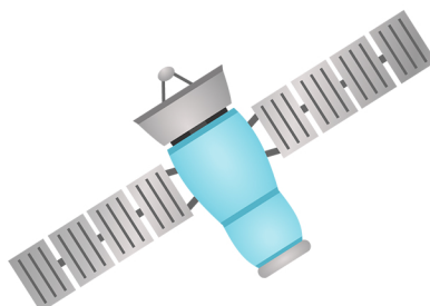
Satelita
