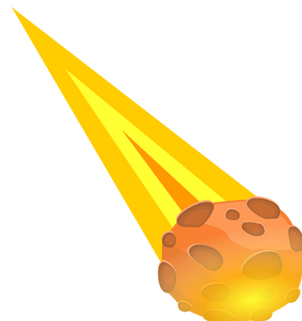
Kometą
