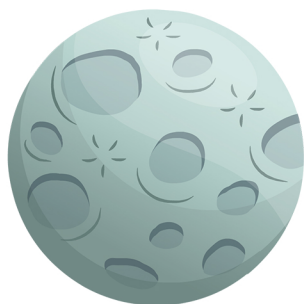
Księżyc
